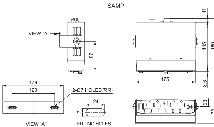
외형도 (단위 : mm)
