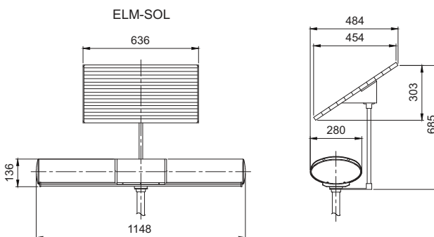
외형도 (단위 : mm)
